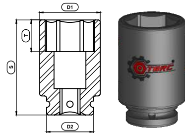
Long Socket
